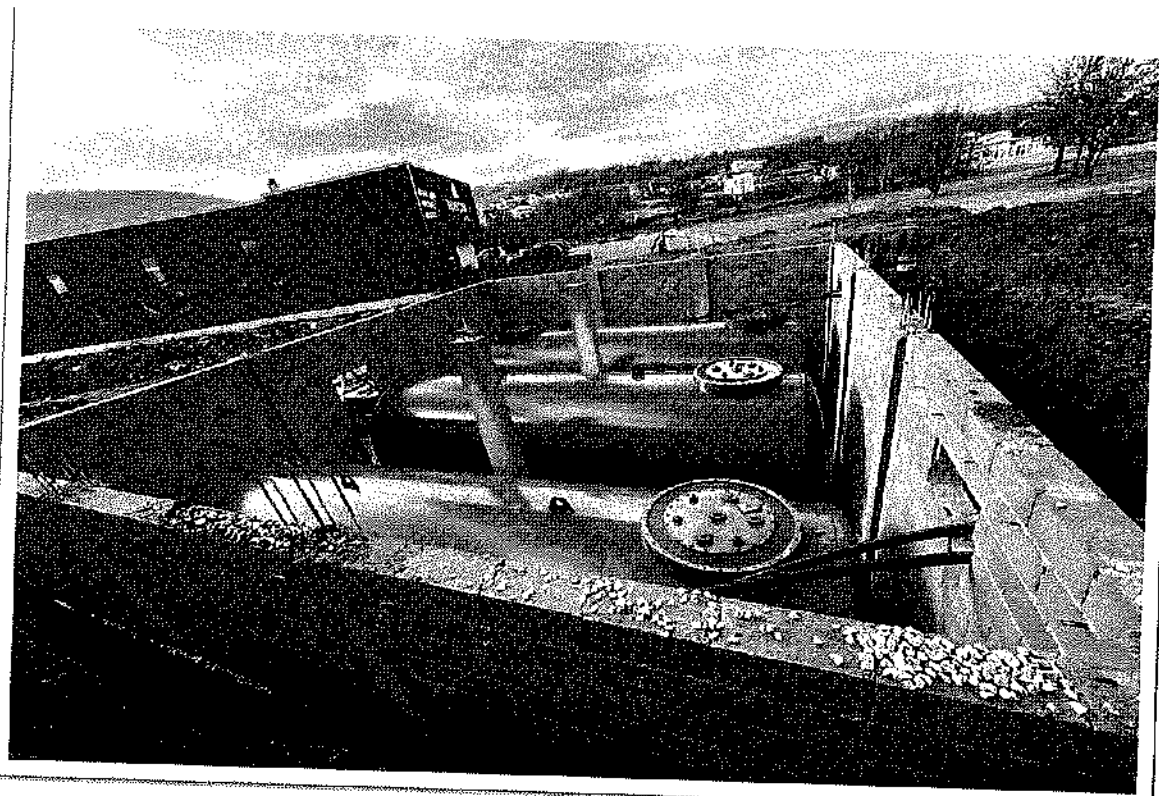
(Foto nr 15 Rezervarët )
