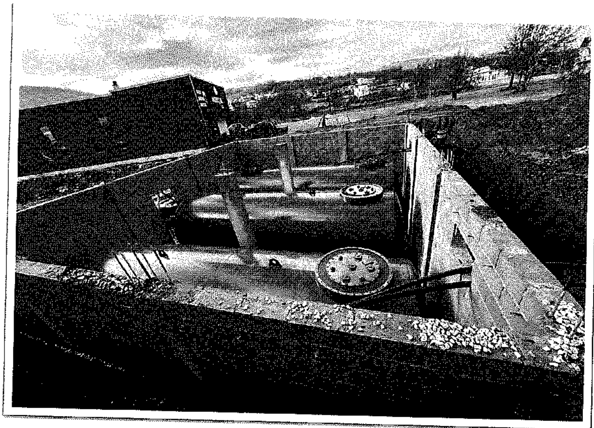
(Foto nr 14 Rezervarët )
